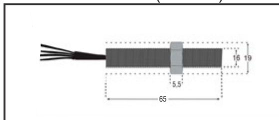
KS3003-B (4 FIOS)
