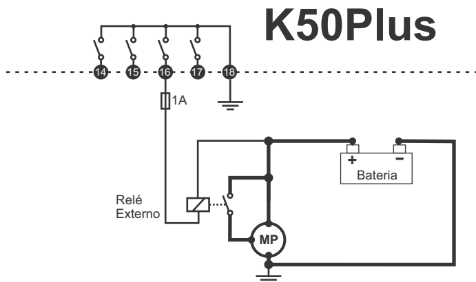
Ligação de relés externos
