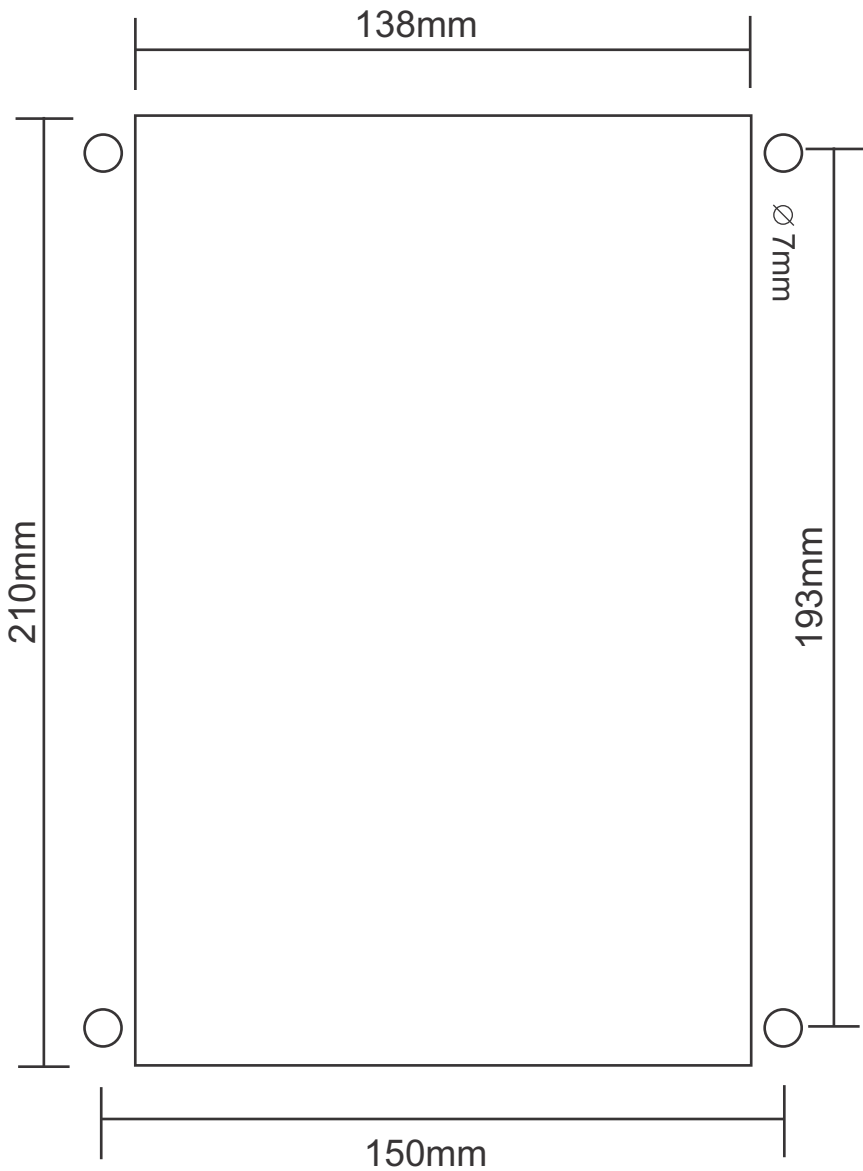
Corte do painel
